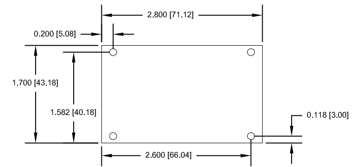
PLITKA 1U 14HP
